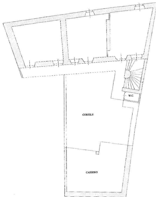
Tav. n. 02/03 PIANTA SCHEMATICA PIANO PRIMO (2° fl.) - scala 1:100
