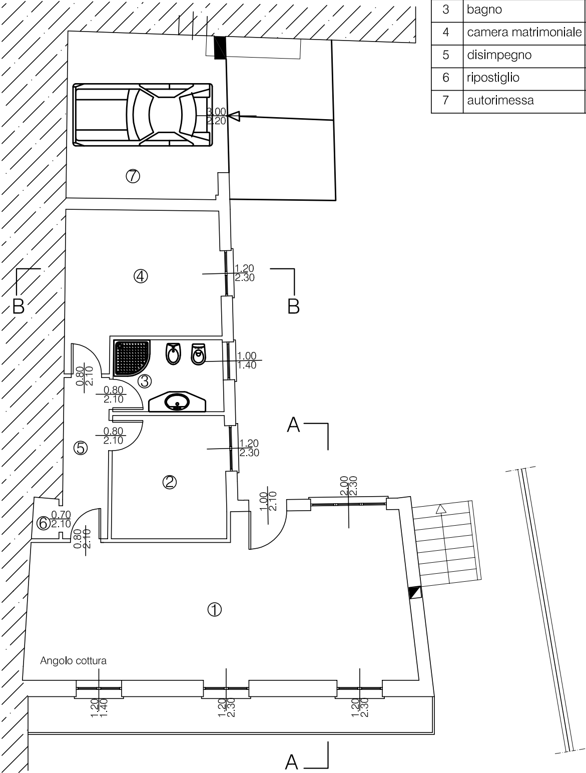
Progetto - Pianta
