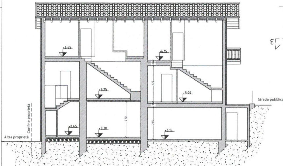
SEZIONE 3-3
