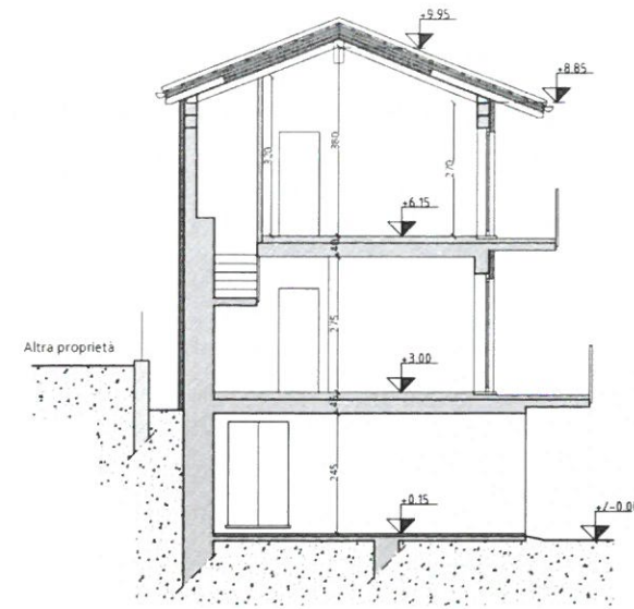
SEZIONE 1-1
