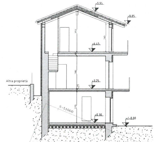
SEZIONE 2-2
