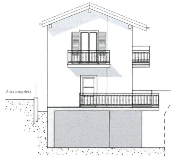
PROSPETTO SUD
