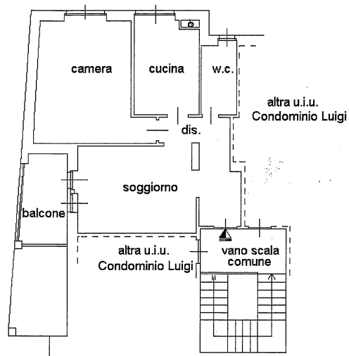
PIANTA PIANO TERZO H=300
