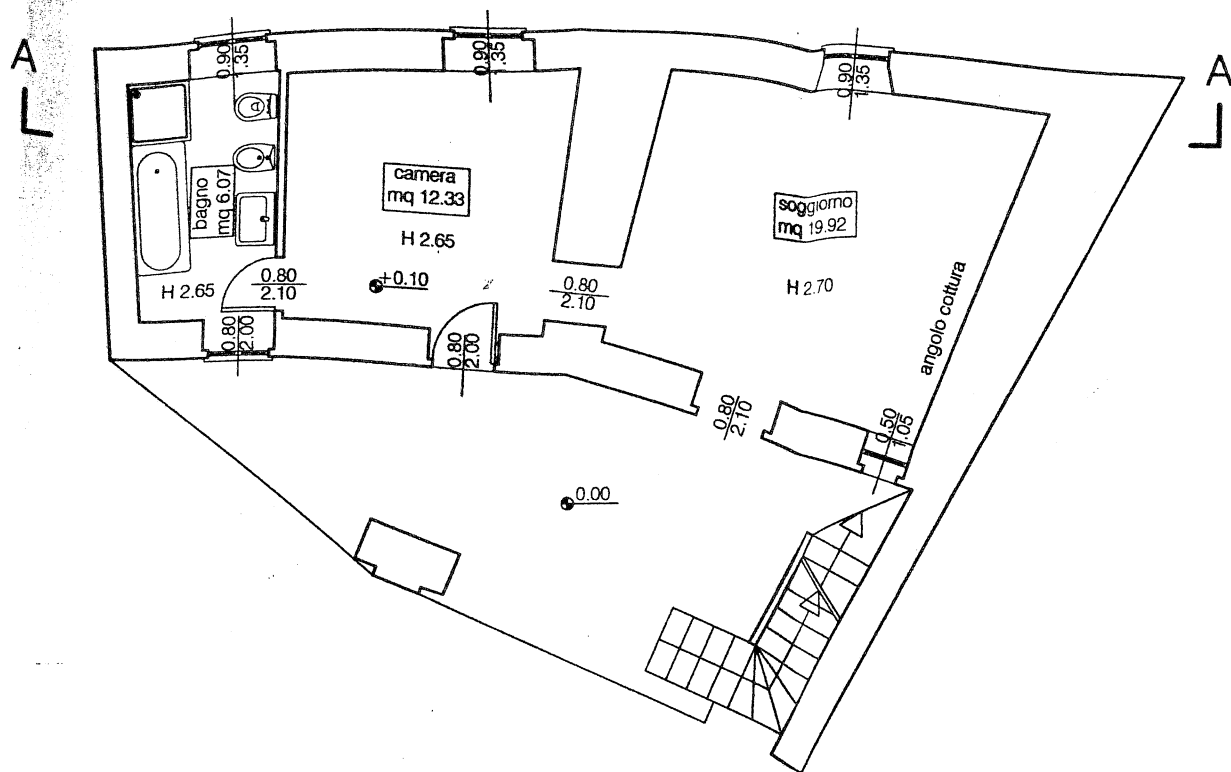
Progetto - Pianta Piano Primo
